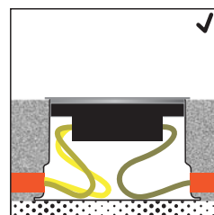
Sænk ned og fastgør.
