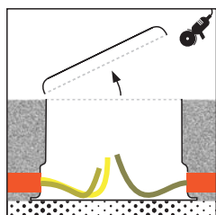
Tilret forskallingens top.
